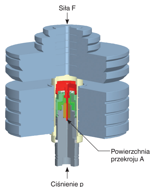
Układ tłokowo-cylindrowy z ciężarkami, z pokrywą
