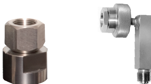
Rys. lewy : przeciwwzłazcze G 3/4 wew. na G 1/2 wew. Rys. prawy: przyłącze kątowe 90°
