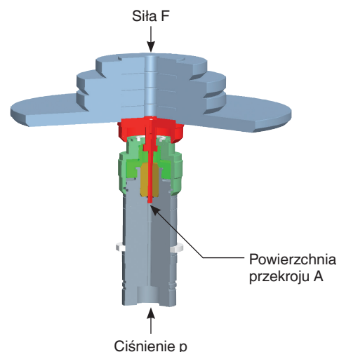
Układ tłokowo-cylindrowy z ciężarkami, bez pokrywy
