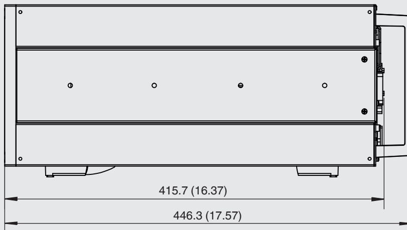
侧视图 (左)
