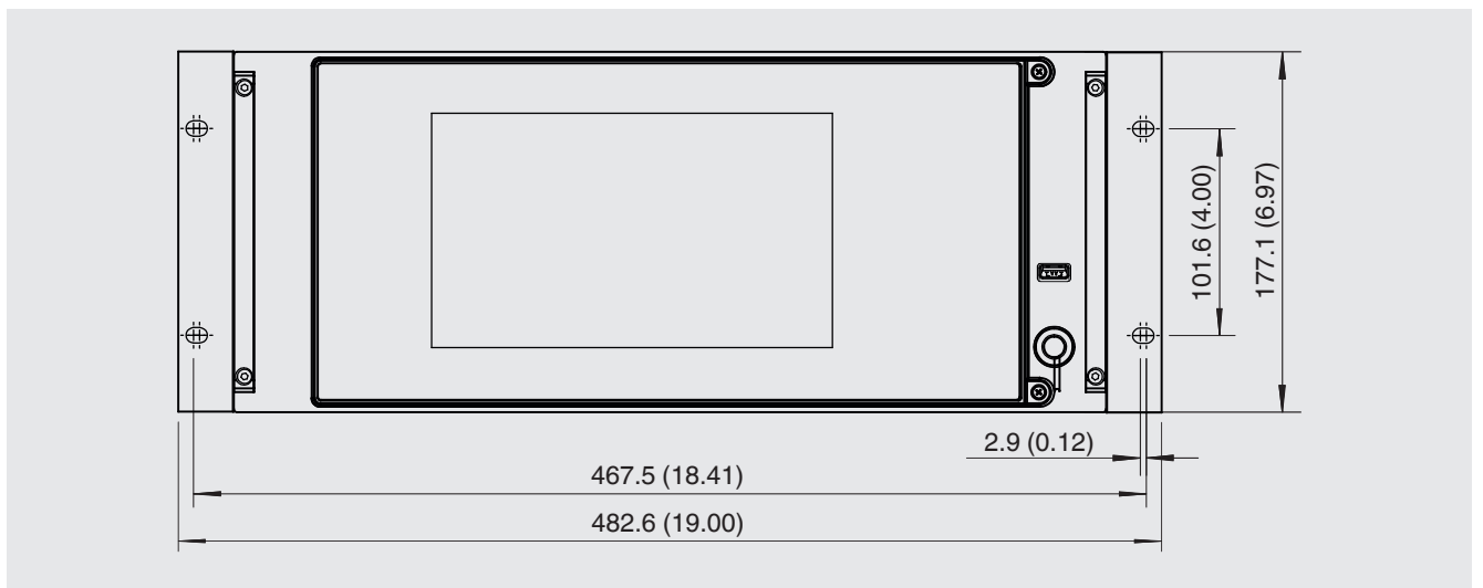
19"机架安装套件 (带侧面板), 正视图
