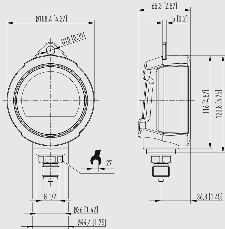
CPG1500 mit Gehäuseschutzkappe
