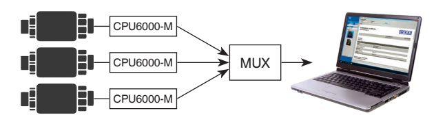
Sensores de presión, multímetros modelo CPU6000-M, multiplexores y ordenador con software WIKa-Cal
