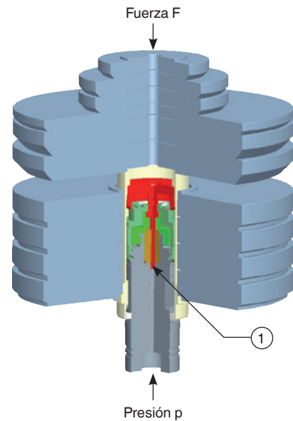
Sistema de pistón-cilindro con pesas y portapesas
