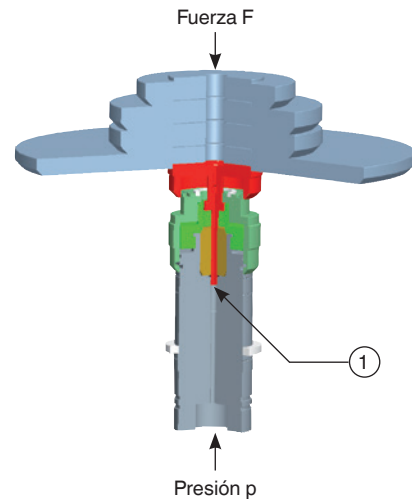
Sistema de pistón-cilindro con pesas sin portapesas
