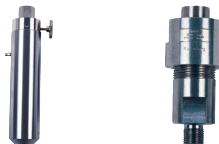
Fig. izquierda: Separador (con membrana) 700 bar (10.000 lb/in 2 )
