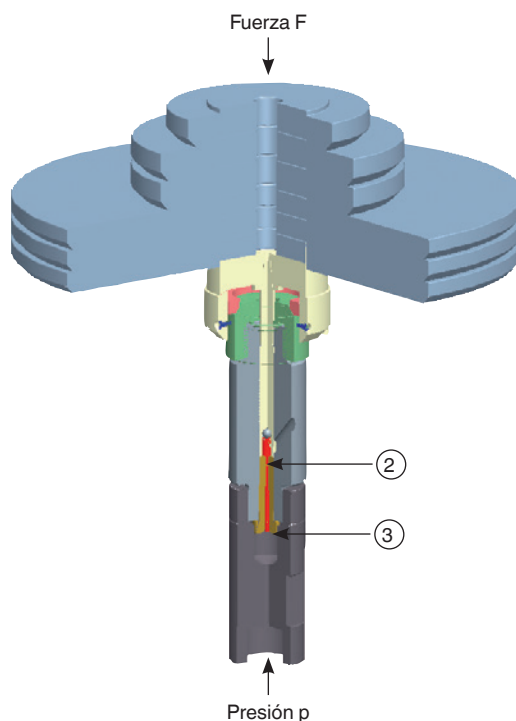
Sistema de pistón-cilindro doble, modelo CPS5800
