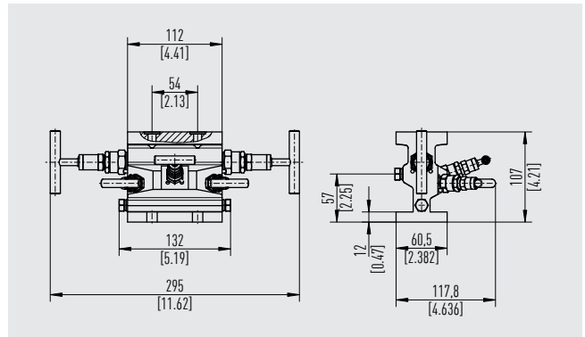
Modello IV52N, forma ad H
