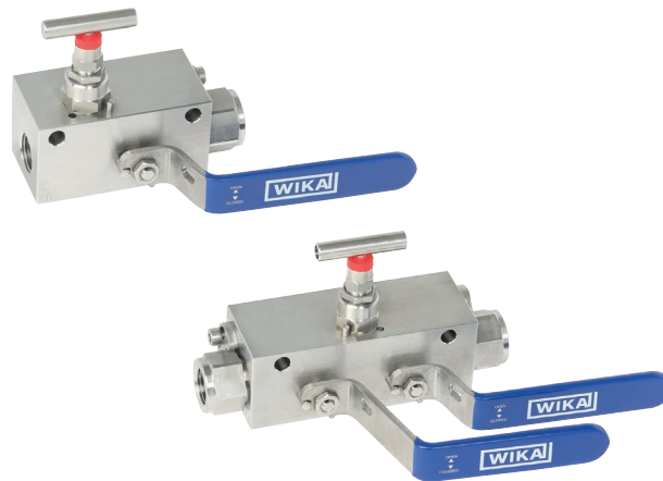
Fig. a sinistra: modello IBM2, valvola di blocco e sfiato Fig. a destra: modello IBM3, doppia valvola di blocco e sfiato
