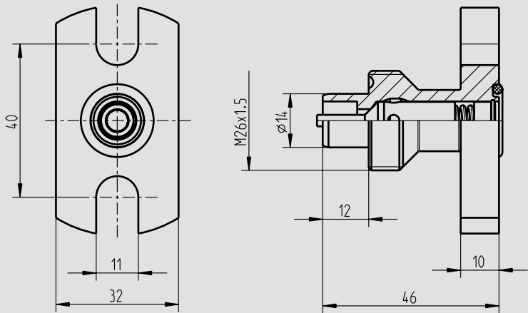
尺寸 (mm)
