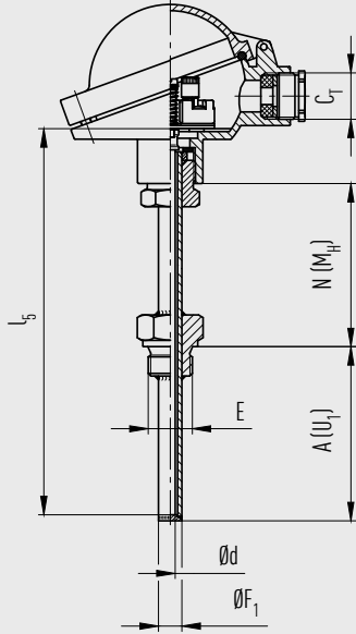
zylindrisches Gewinde
