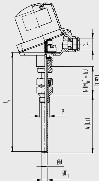
zylindrisches Gewinde
