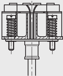
Messeinsatz mit aufgebautem Transmitter
