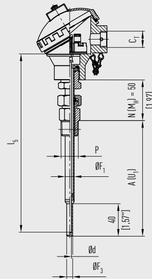
kegeliges Gewinde
