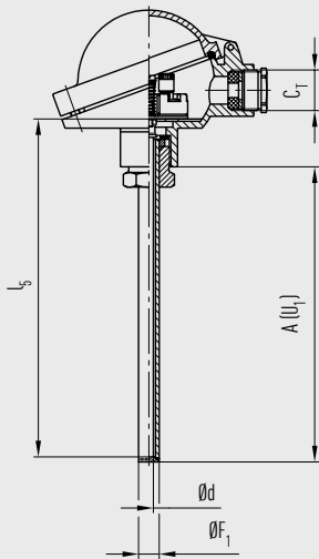
ohne Gewinde (glatt)
