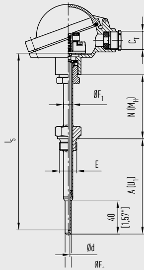
zylindrisches Gewinde
