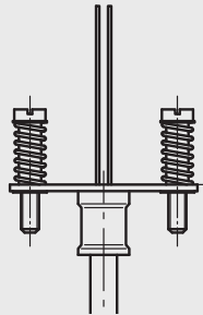
Messeinsatz vorbereitet für Transmittermontage
