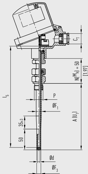
zylindrisches Gewinde
