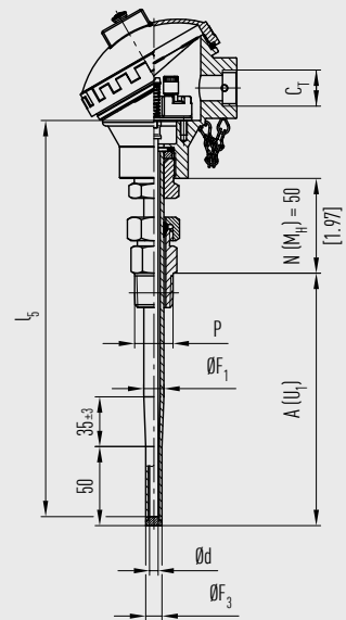
kegeliges Gewinde
