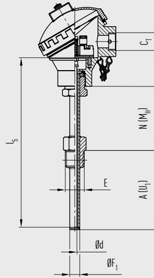
kegeliges Gewinde
