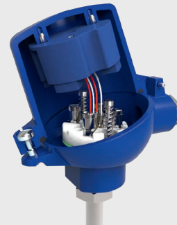
Montage im Deckel des Anschlusskopfs
