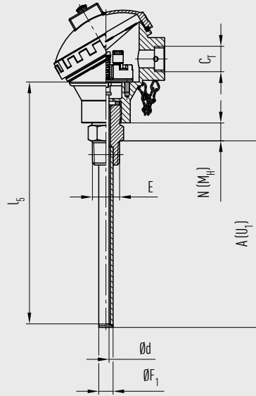
kegeliges Gewinde
