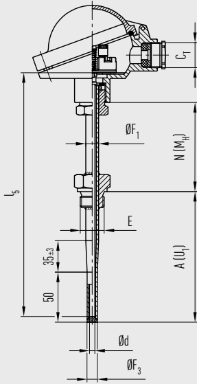
zylindrisches Gewinde
