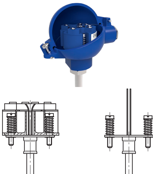
Abb. links: Messeinsatz mit aufgebautem Transmitter (hier: Typ T32) Abb. rechts: Messeinsatz vorbereitet für Transmittermontage
