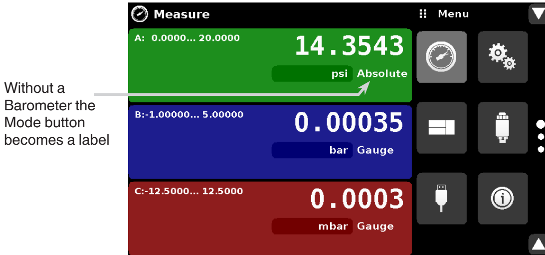
Figure 6.4.1.1-A - Mode Label
