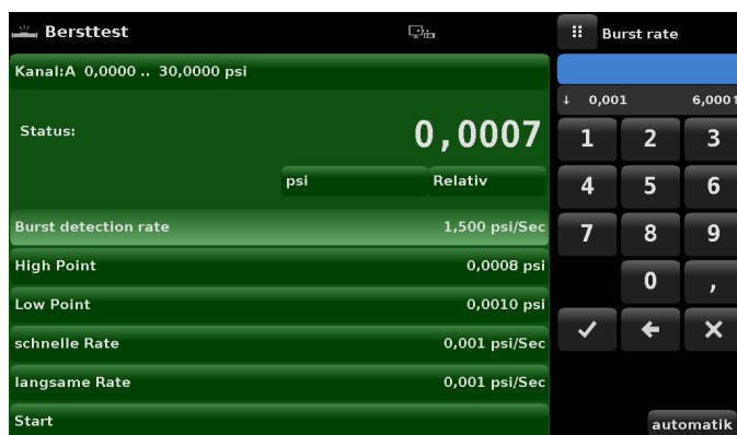
Abb. 6.4.14-B - Bersterkennungsrate
