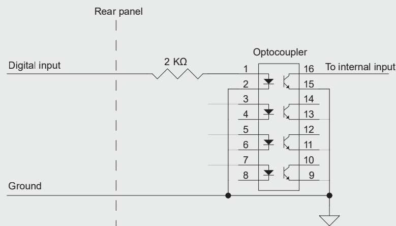
Abb. 7.1.1.1-A - Schaltplan Digitaleingang
