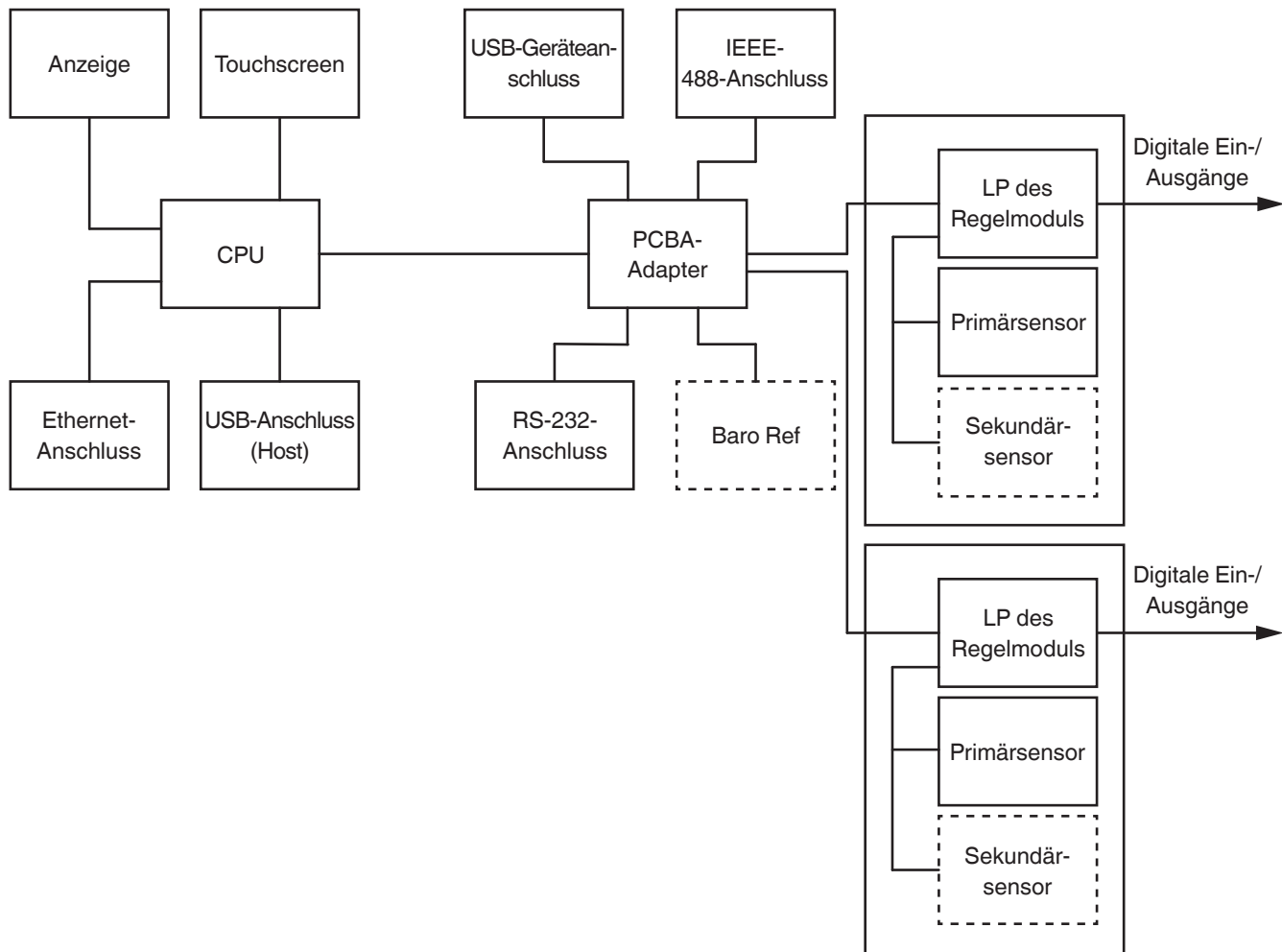
Abb. 3.6 - Elektrisches Blockschaltbild
