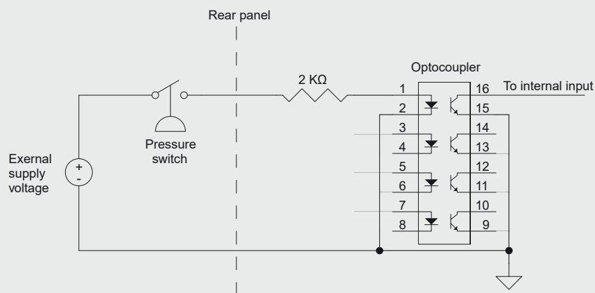
Abb. 7.1.1.1-C - Digitaleingang mit Druckschalter
