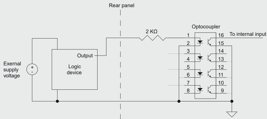
Abb. 7.1.1.1-B - Digitaleingang mit Logikbaustein
