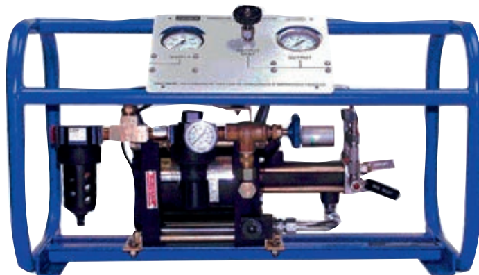
Abb. 8.12 – Druckverdichter Typ 75
