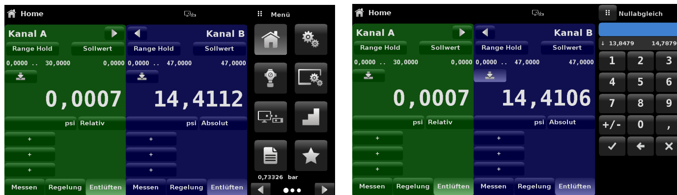
Abb. 6.4.1.6 - Nullpunktabgleich, relativ - absolut
