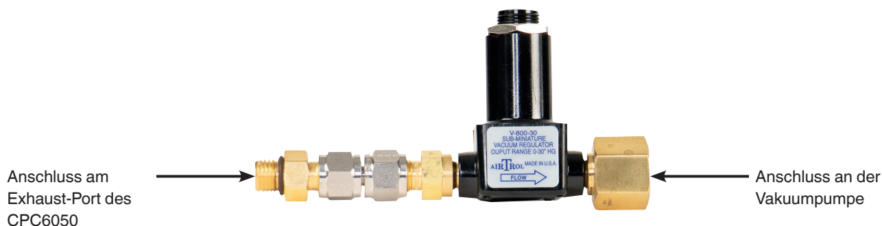
Abb. 8.11-B - Vakuumregler
